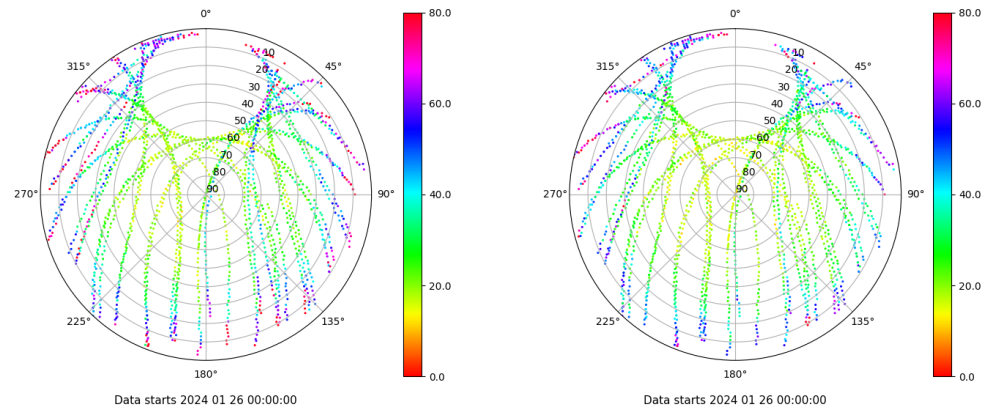
Skyplot for station VIGO. Parameter M1C Data file VIGO00ESP_R_2024026.xtr Skyplot for station VIGO. Parameter M2C Data file VIGO00ESP_R_2024026.xtr
