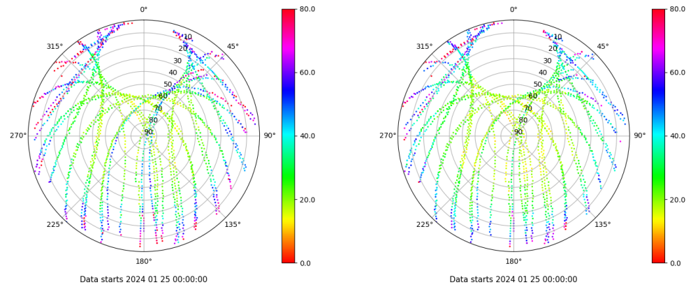
Skyplot for station VIGO. Parameter M1C Data file VIGO00ESP_R_2024025.xtr Skyplot for station VIGO. Parameter M2C Data file VIGO00ESP_R_2024025.xtr
