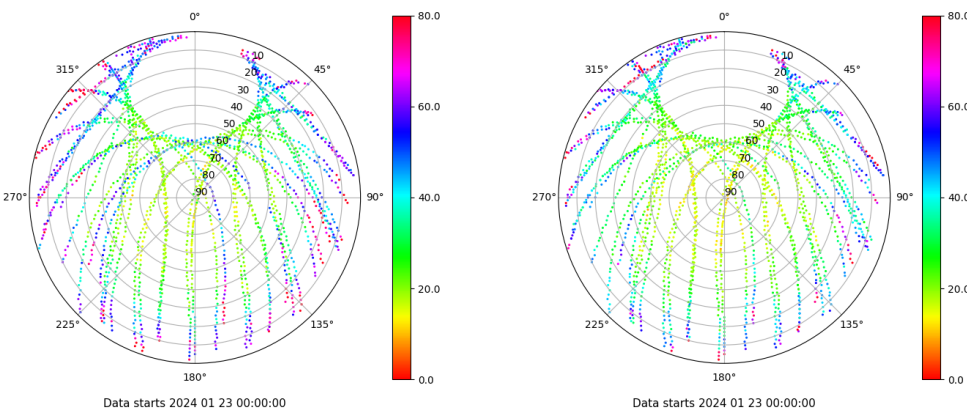
Skyplot for station VIGO. Parameter M1C Data file VIGO00ESP_R_2024023.xtr Skyplot for station VIGO. Parameter M2C Data file VIGO00ESP_R_2024023.xtr
