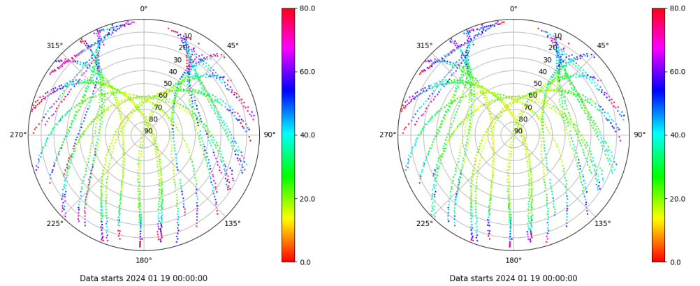
Skyplot for station VIGO. Parameter M1C Data file VIGO00ESP_R_2024019.xtr Skyplot for station VIGO. Parameter M2C Data file VIGO00ESP_R_2024019.xtr
