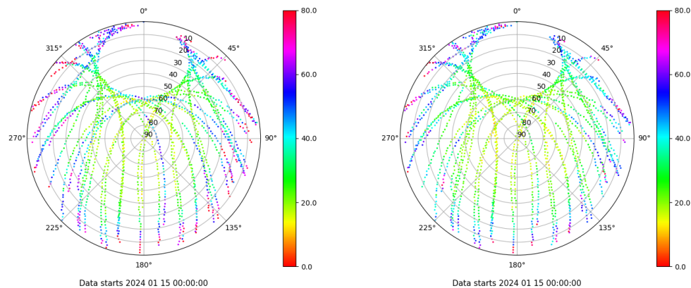
Skyplot for station VIGO. Parameter M1C Data file VIGO00ESP_R_2024015.xtr Skyplot for station VIGO. Parameter M2C Data file VIGO00ESP_R_2024015.xtr
