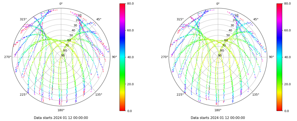
Skyplot for station VIGO. Parameter M1C Data file VIGO00ESP_R_2024012.xtr Skyplot for station VIGO. Parameter M2C Data file VIGO00ESP_R_2024012.xtr
