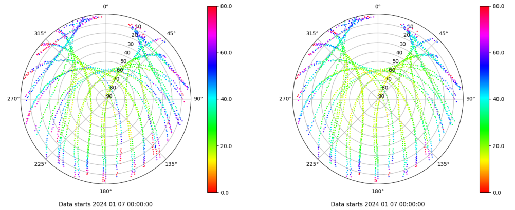
Skyplot for station VIGO. Parameter M1C Data file VIGO00ESP_R_2024007.xtr Skyplot for station VIGO. Parameter M2C Data file VIGO00ESP_R_2024007.xtr
