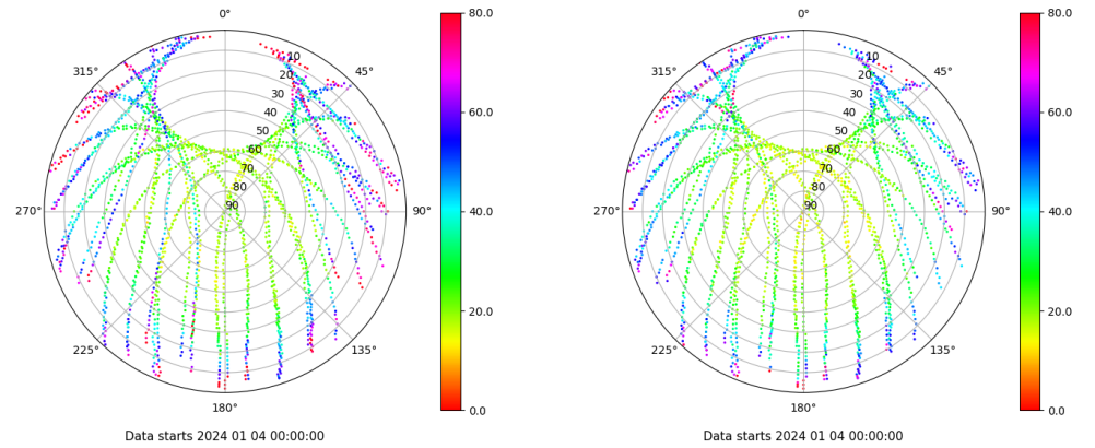
Skyplot for station VIGO. Parameter M1C Data file VIGO00ESP_R_2024004.xtr Skyplot for station VIGO. Parameter M2C Data file VIGO00ESP_R_2024004.xtr
