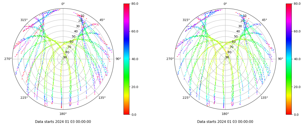
Skyplot for station VIGO. Parameter M1C Data file VIGO00ESP_R_2024003.xtr Skyplot for station VIGO. Parameter M2C Data file VIGO00ESP_R_2024003.xtr
