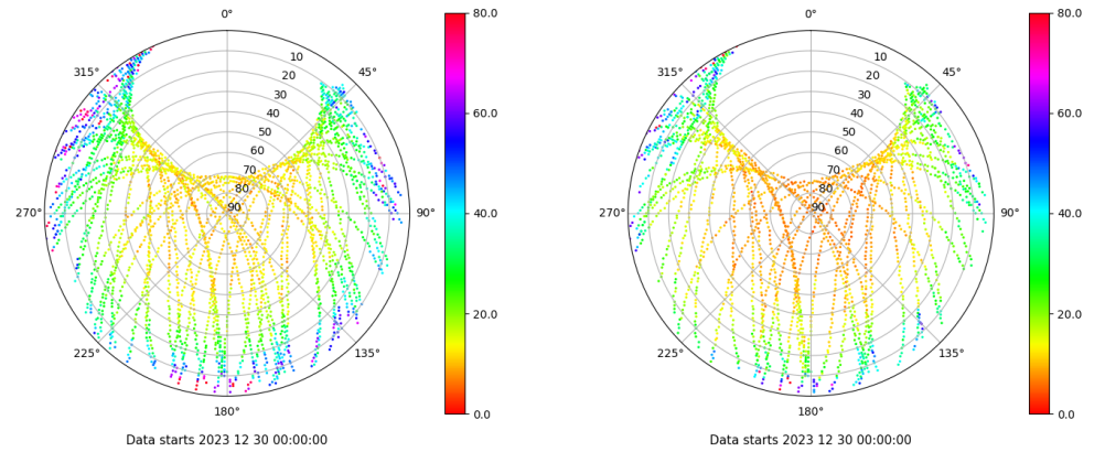
Skyplot for station VIGO. Parameter M1C Data file VIGO00ESP_R_2023364.xtr Skyplot for station VIGO. Parameter M2X Data file VIGO00ESP_R_2023364.xtr
