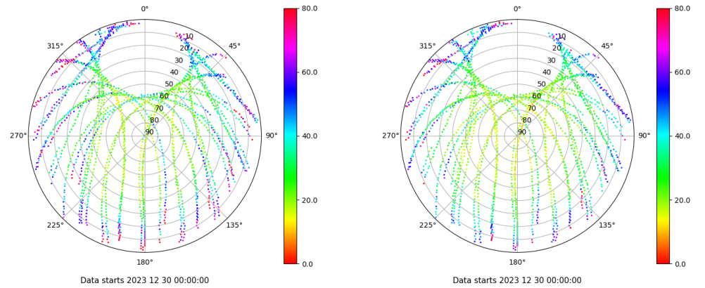
Skyplot for station VIGO. Parameter M1C Data file VIGO00ESP_R_2023364.xtr Skyplot for station VIGO. Parameter M2C Data file VIGO00ESP_R_2023364.xtr
