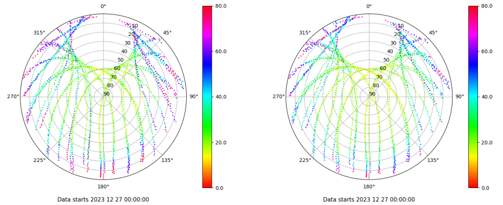
Skyplot for station VIGO. Parameter M1C Data file VIGO00ESP_R_2023361.xtr Skyplot for station VIGO. Parameter M2C Data file VIGO00ESP_R_2023361.xtr
