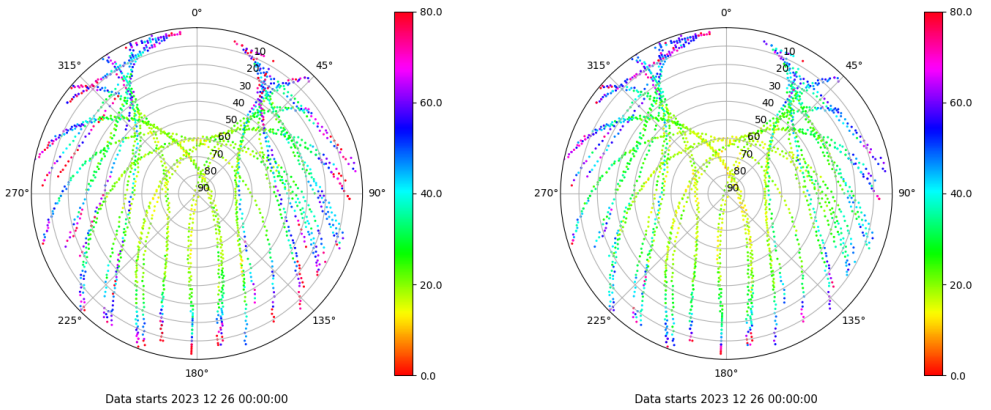
Skyplot for station VIGO. Parameter M1C Data file VIGO00ESP_R_2023360.xtr Skyplot for station VIGO. Parameter M2C Data file VIGO00ESP_R_2023360.xtr
