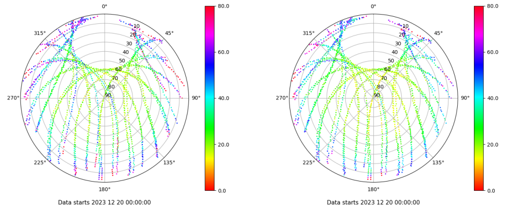
Skyplot for station VIGO. Parameter M1C Data file VIGO00ESP_R_2023354.xtr Skyplot for station VIGO. Parameter M2C Data file VIGO00ESP_R_2023354.xtr
