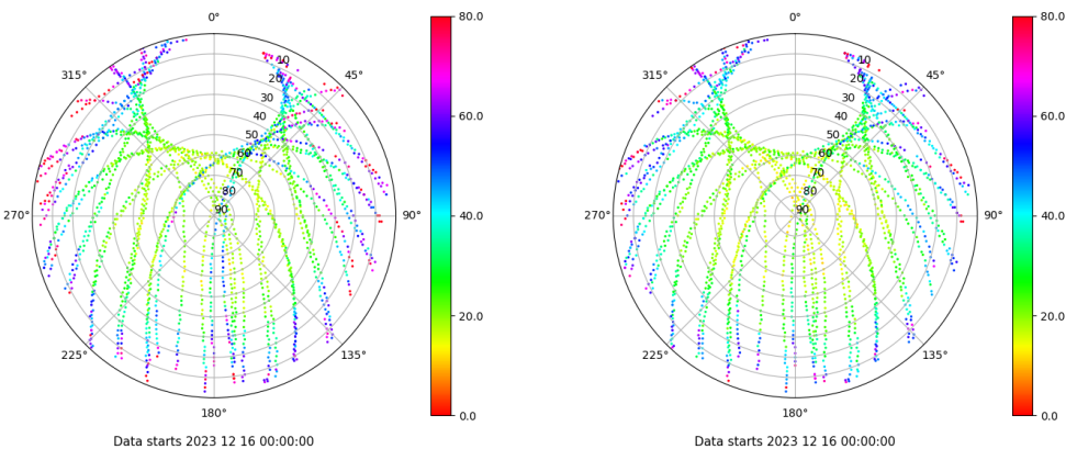
Skyplot for station VIGO. Parameter M1C Data file VIGO00ESP_R_2023350.xtr Skyplot for station VIGO. Parameter M2C Data file VIGO00ESP_R_2023350.xtr
