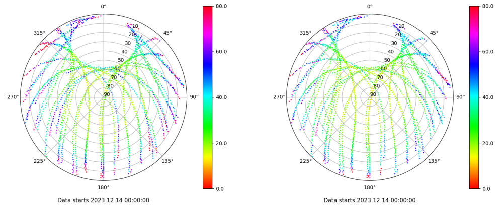
Skyplot for station VIGO. Parameter M1C Data file VIGO00ESP_R_2023348.xtr Skyplot for station VIGO. Parameter M2C Data file VIGO00ESP_R_2023348.xtr
