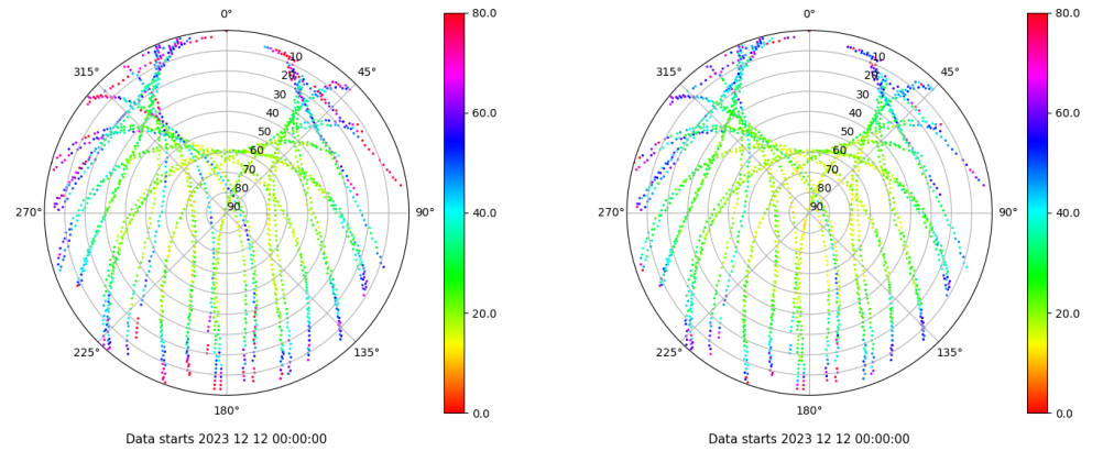
Skyplot for station VIGO. Parameter M1C Data file VIGO00ESP_R_2023346.xtr Skyplot for station VIGO. Parameter M2C Data file VIGO00ESP_R_2023346.xtr
