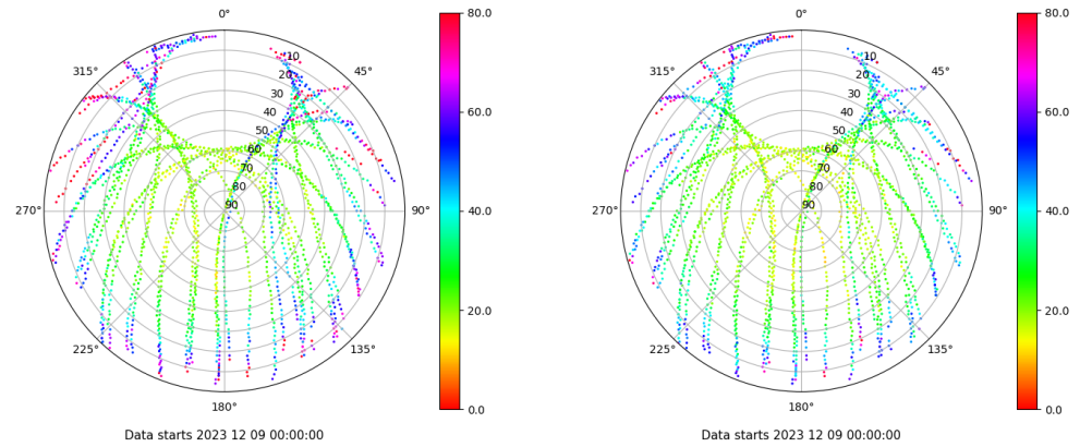
Skyplot for station VIGO. Parameter M1C Data file VIGO00ESP_R_2023343.xtr Skyplot for station VIGO. Parameter M2C Data file VIGO00ESP_R_2023343.xtr
