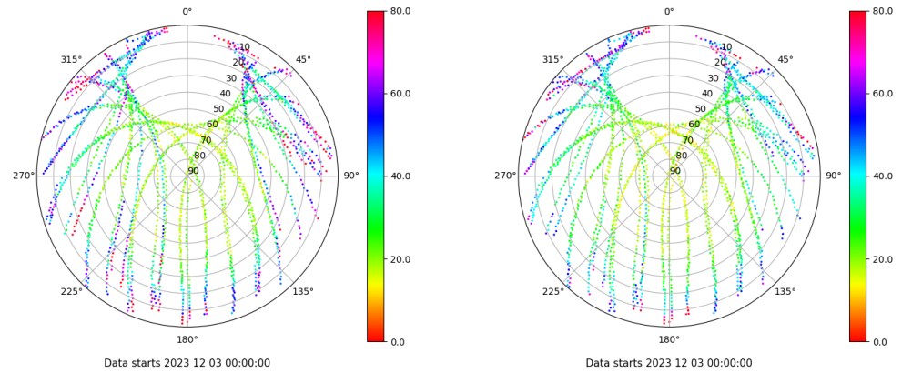
Skyplot for station VIGO. Parameter M1C Data file VIGO00ESP_R_2023337.xtr Skyplot for station VIGO. Parameter M2C Data file VIGO00ESP_R_2023337.xtr
