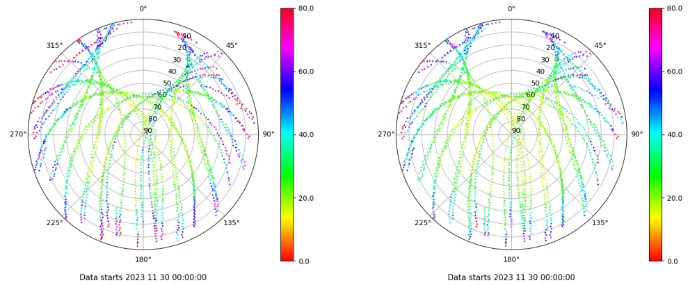
Skyplot for station VIGO. Parameter M1C Data file VIGO00ESP_R_2023334.xtr Skyplot for station VIGO. Parameter M2C Data file VIGO00ESP_R_2023334.xtr
