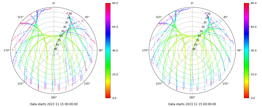
Skyplot for station VIGO. Parameter M1C Data file VIGO00ESP_R_2023319.xtr Skyplot for station VIGO. Parameter M2C Data file VIGO00ESP_R_2023319.xtr
