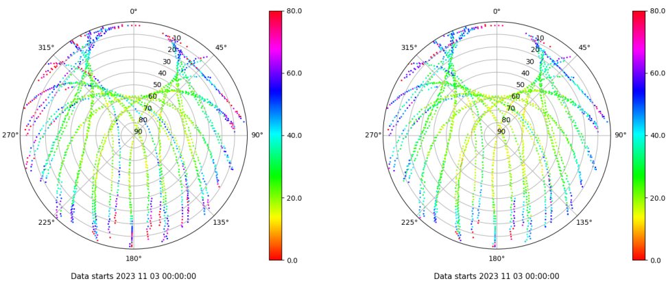
Skyplot for station VIGO. Parameter M1C Data file VIGO00ESP_R_2023307.xtr Skyplot for station VIGO. Parameter M2C Data file VIGO00ESP_R_2023307.xtr
