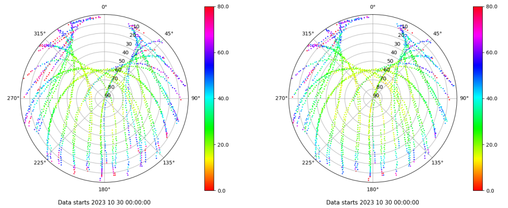
Skyplot for station VIGO. Parameter M1C Data file VIGO00ESP_R_2023303.xtr Skyplot for station VIGO. Parameter M2C Data file VIGO00ESP_R_2023303.xtr
