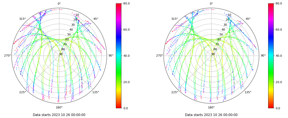
Skyplot for station VIGO. Parameter M1C Data file VIGO00ESP_R_2023299.xtr Skyplot for station VIGO. Parameter M2C Data file VIGO00ESP_R_2023299.xtr
