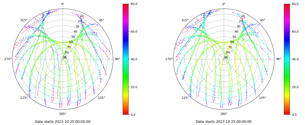
Skyplot for station VIGO. Parameter M1C Data file VIGO00ESP_R_2023298.xtr Skyplot for station VIGO. Parameter M2C Data file VIGO00ESP_R_2023298.xtr
