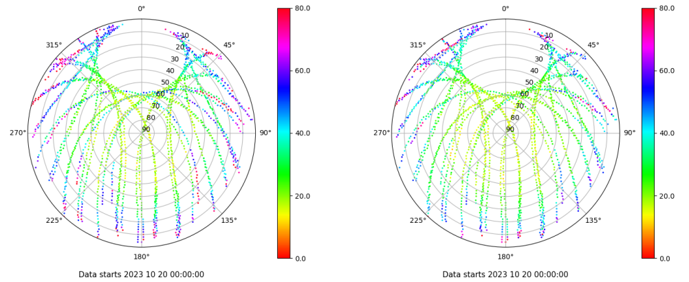
Skyplot for station VIGO. Parameter M1C Data file VIGO00ESP_R_2023293.xtr Skyplot for station VIGO. Parameter M2C Data file VIGO00ESP_R_2023293.xtr
