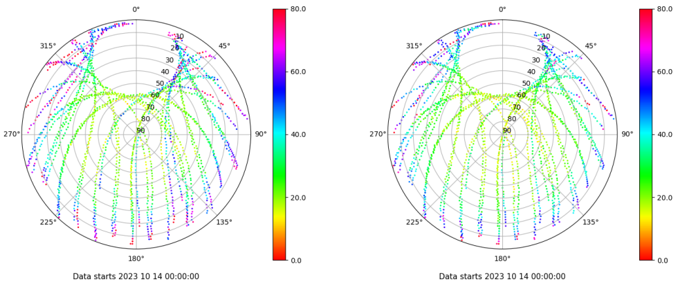
Skyplot for station VIGO. Parameter M1C Data file VIGO00ESP_R_2023287.xtr Skyplot for station VIGO. Parameter M2C Data file VIGO00ESP_R_2023287.xtr
