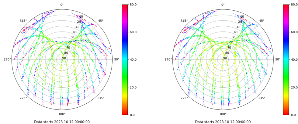
Skyplot for station VIGO. Parameter M1C Data file VIGO00ESP_R_2023285.xtr Skyplot for station VIGO. Parameter M2C Data file VIGO00ESP_R_2023285.xtr
