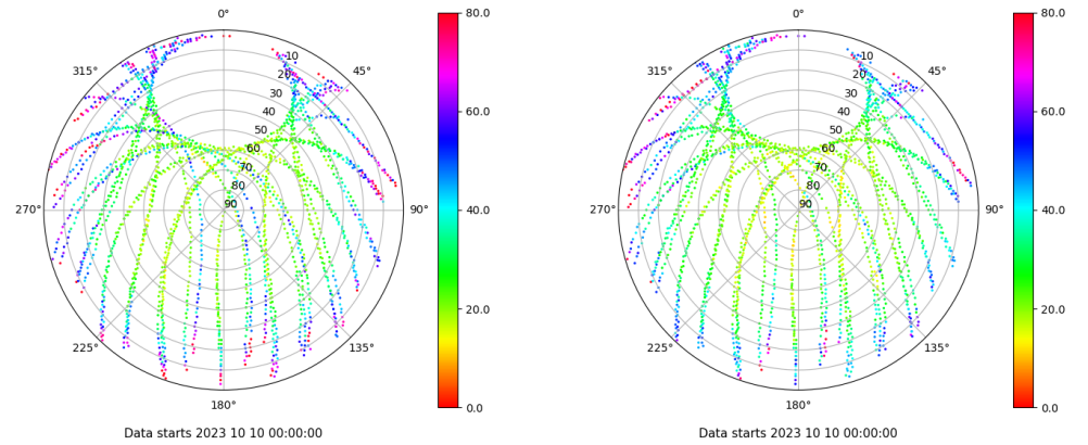
Skyplot for station VIGO. Parameter M1C Data file VIGO00ESP_R_2023283.xtr Skyplot for station VIGO. Parameter M2C Data file VIGO00ESP_R_2023283.xtr
