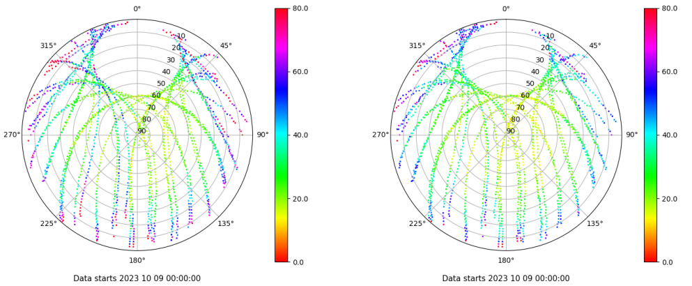
Skyplot for station VIGO. Parameter M1C Data file VIGO00ESP_R_2023282.xtr Skyplot for station VIGO. Parameter M2C Data file VIGO00ESP_R_2023282.xtr
