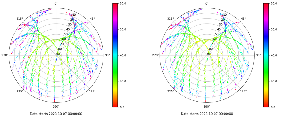
Skyplot for station VIGO. Parameter M1C Data file VIGO00ESP_R_2023280.xtr Skyplot for station VIGO. Parameter M2C Data file VIGO00ESP_R_2023280.xtr
