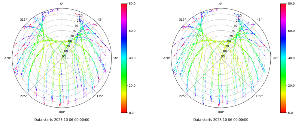
Skyplot for station VIGO. Parameter M1C Data file VIGO00ESP_R_2023279.xtr Skyplot for station VIGO. Parameter M2C Data file VIGO00ESP_R_2023279.xtr
