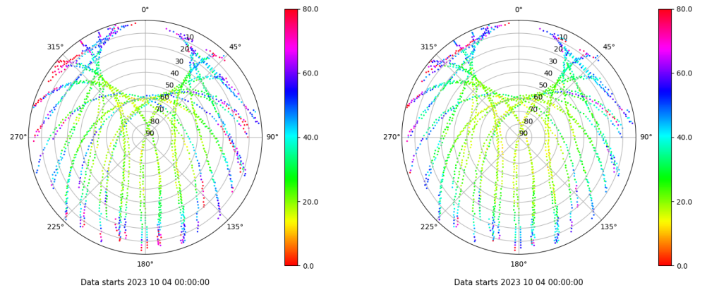
Skyplot for station VIGO. Parameter M1C Data file VIGO00ESP_R_2023277.xtr Skyplot for station VIGO. Parameter M2C Data file VIGO00ESP_R_2023277.xtr
