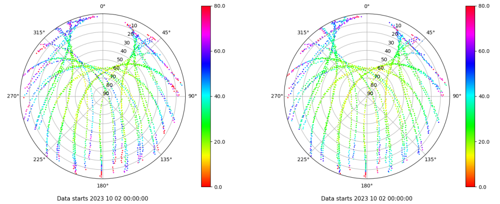
Skyplot for station VIGO. Parameter M1C Data file VIGO00ESP_R_2023275.xtr Skyplot for station VIGO. Parameter M2C Data file VIGO00ESP_R_2023275.xtr
