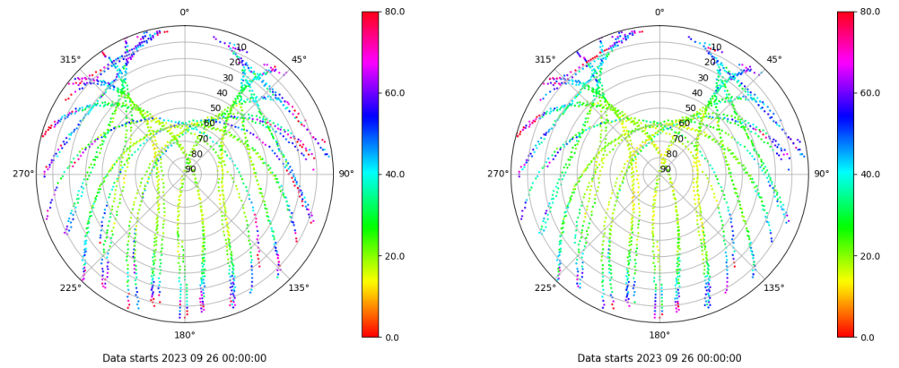
Skyplot for station VIGO. Parameter M1C Data file VIGO00ESP_R_2023269.xtr Skyplot for station VIGO. Parameter M2C Data file VIGO00ESP_R_2023269.xtr
