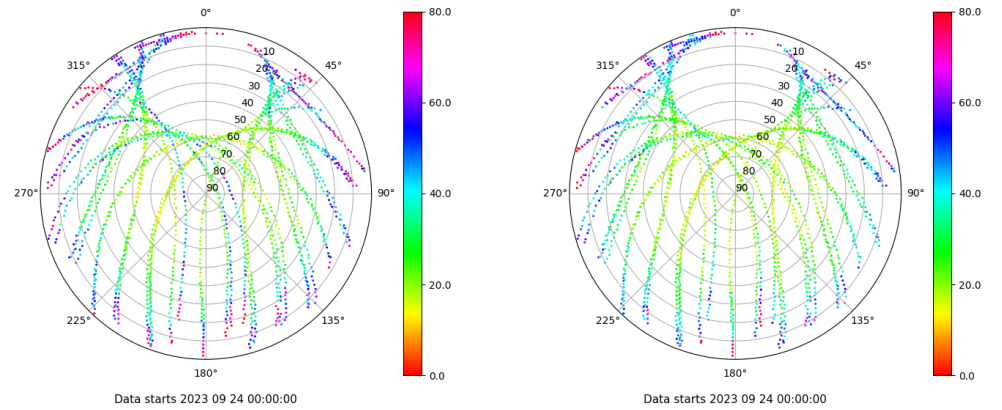
Skyplot for station VIGO. Parameter M1C Data file VIGO00ESP_R_2023267.xtr Skyplot for station VIGO. Parameter M2C Data file VIGO00ESP_R_2023267.xtr
