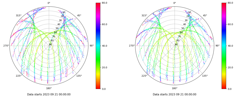
Skyplot for station VIGO. Parameter M1C Data file VIGO00ESP_R_2023264.xtr Skyplot for station VIGO. Parameter M2C Data file VIGO00ESP_R_2023264.xtr
