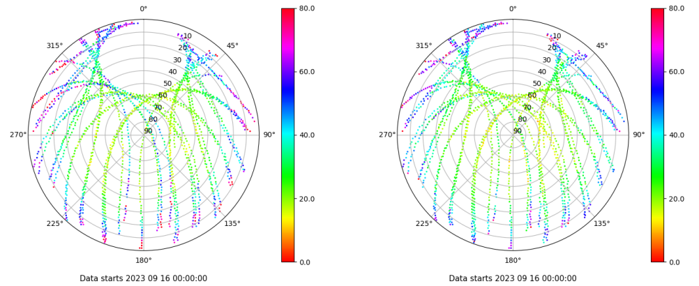
Skyplot for station VIGO. Parameter M1C Data file VIGO00ESP_R_2023259.xtr Skyplot for station VIGO. Parameter M2C Data file VIGO00ESP_R_2023259.xtr
