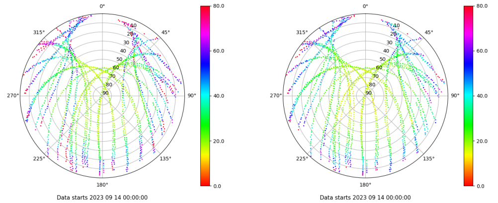
Skyplot for station VIGO. Parameter M1C Data file VIGO00ESP_R_2023257.xtr Skyplot for station VIGO. Parameter M2C Data file VIGO00ESP_R_2023257.xtr
