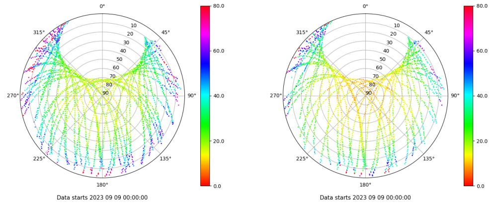
Skyplot for station VIGO. Parameter M1C Data file VIGO00ESP_R_2023252.xtr Skyplot for station VIGO. Parameter M2X Data file VIGO00ESP_R_2023252.xtr
