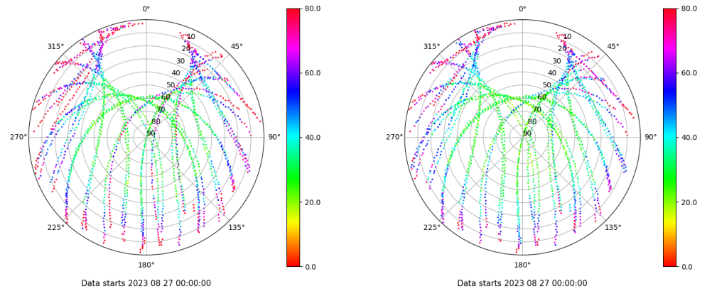
Skyplot for station VIGO. Parameter M1C Data file VIGO00ESP_R_2023239.xtr Skyplot for station VIGO. Parameter M2C Data file VIGO00ESP_R_2023239.xtr
