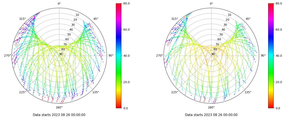
Skyplot for station VIGO. Parameter M1C Data file VIGO00ESP_R_2023238.xtr Skyplot for station VIGO. Parameter M2X Data file VIGO00ESP_R_2023238.xtr
