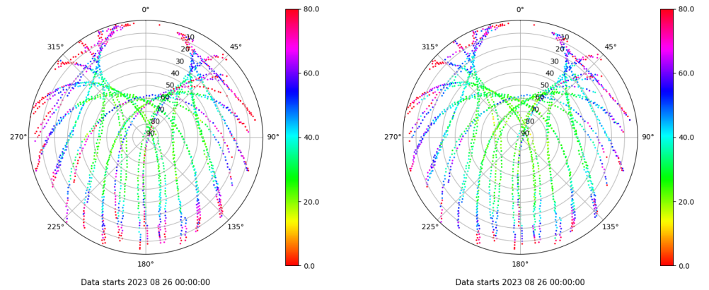
Skyplot for station VIGO. Parameter M1C Data file VIGO00ESP_R_2023238.xtr Skyplot for station VIGO. Parameter M2C Data file VIGO00ESP_R_2023238.xtr
