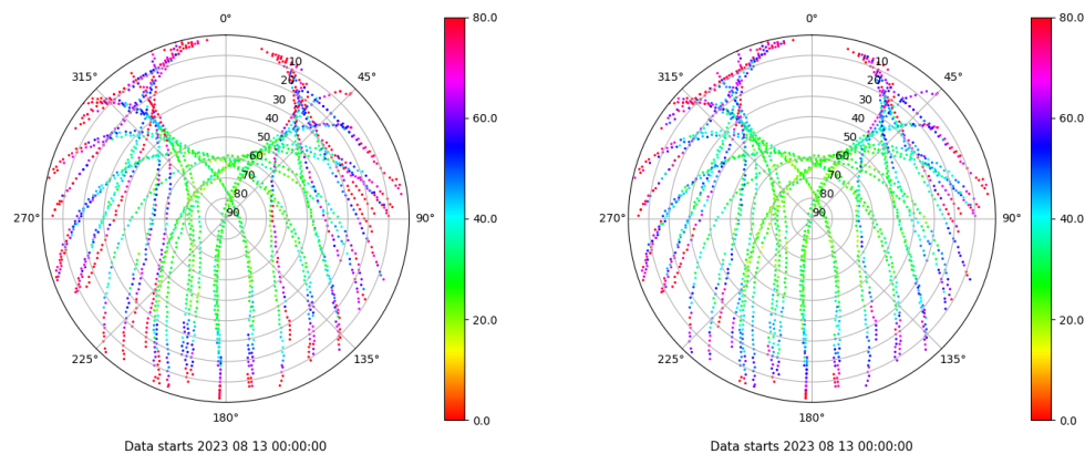
Skyplot for station VIGO. Parameter M1C Data file VIGO00ESP_R_2023225.xtr Skyplot for station VIGO. Parameter M2C Data file VIGO00ESP_R_2023225.xtr
