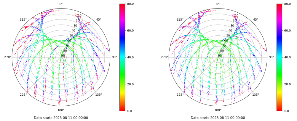
Skyplot for station VIGO. Parameter M1C Data file VIGO00ESP_R_2023223.xtr Skyplot for station VIGO. Parameter M2C Data file VIGO00ESP_R_2023223.xtr
