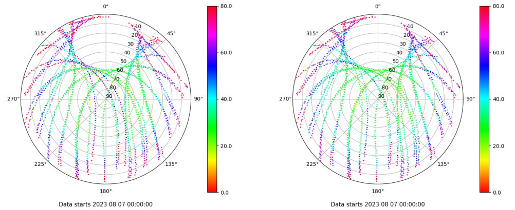
Skyplot for station VIGO. Parameter M1C Data file VIGO00ESP_R_2023219.xtr Skyplot for station VIGO. Parameter M2C Data file VIGO00ESP_R_2023219.xtr
