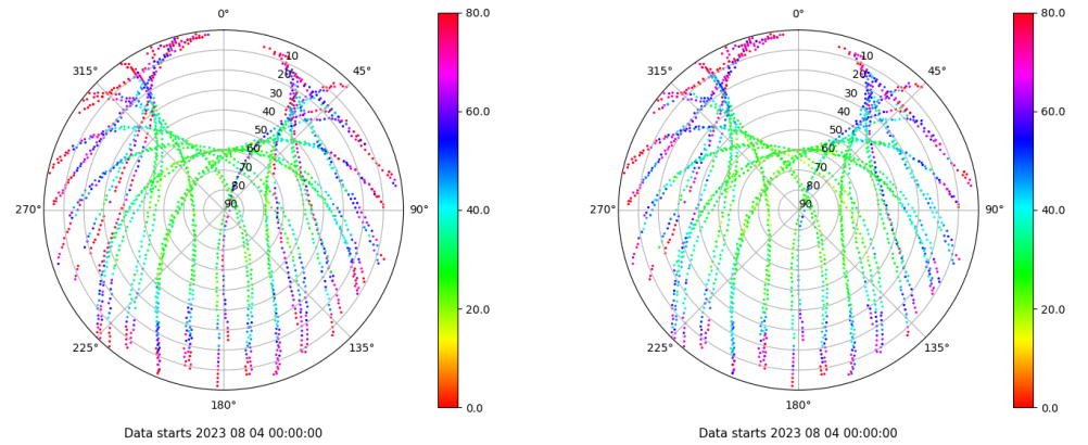
Skyplot for station VIGO. Parameter M1C Data file VIGO00ESP_R_2023216.xtr Skyplot for station VIGO. Parameter M2C Data file VIGO00ESP_R_2023216.xtr
