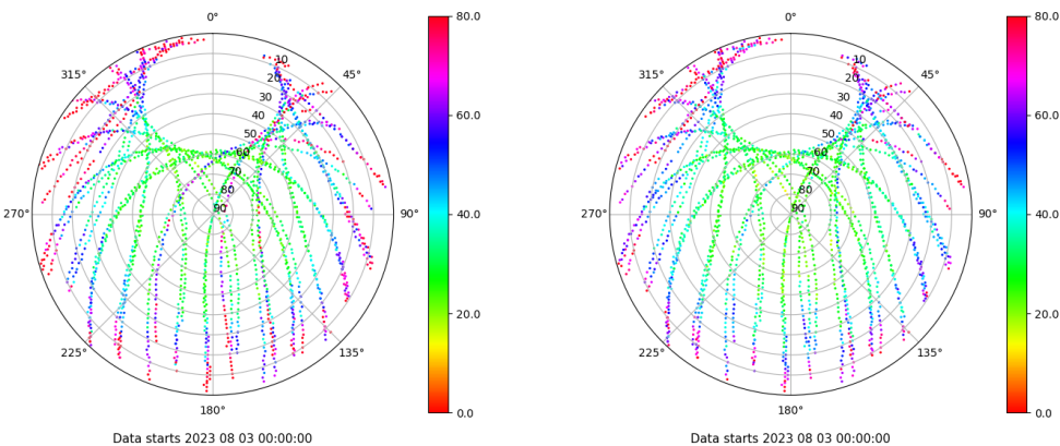
Skyplot for station VIGO. Parameter M1C Data file VIGO00ESP_R_2023215.xtr Skyplot for station VIGO. Parameter M2C Data file VIGO00ESP_R_2023215.xtr
