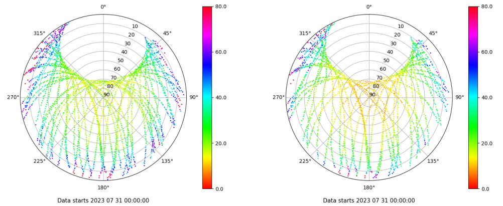
Skyplot for station VIGO. Parameter M1C Data file VIGO00ESP_R_2023212.xtr Skyplot for station VIGO. Parameter M2X Data file VIGO00ESP_R_2023212.xtr
