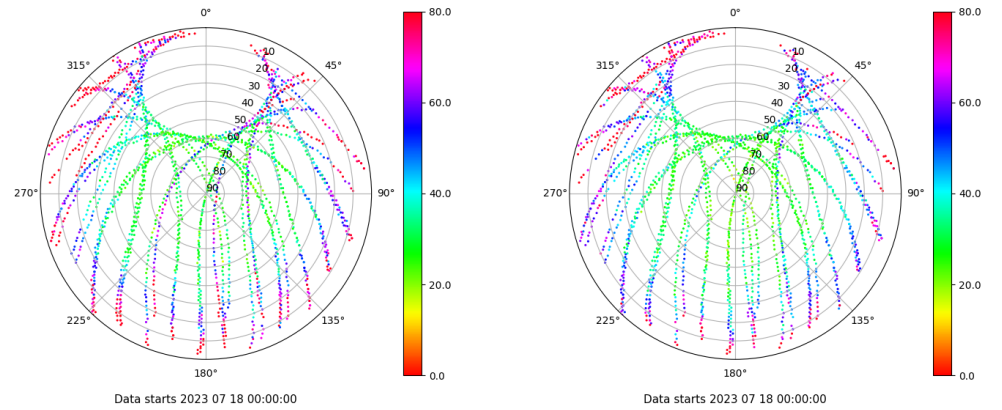
Skyplot for station VIGO. Parameter M1C Data file VIGO00ESP_R_2023199.xtr Skyplot for station VIGO. Parameter M2C Data file VIGO00ESP_R_2023199.xtr
