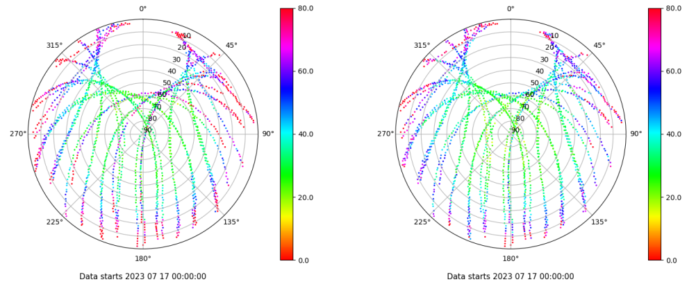
Skyplot for station VIGO. Parameter M1C Data file VIGO00ESP_R_2023198.xtr Skyplot for station VIGO. Parameter M2C Data file VIGO00ESP_R_2023198.xtr
