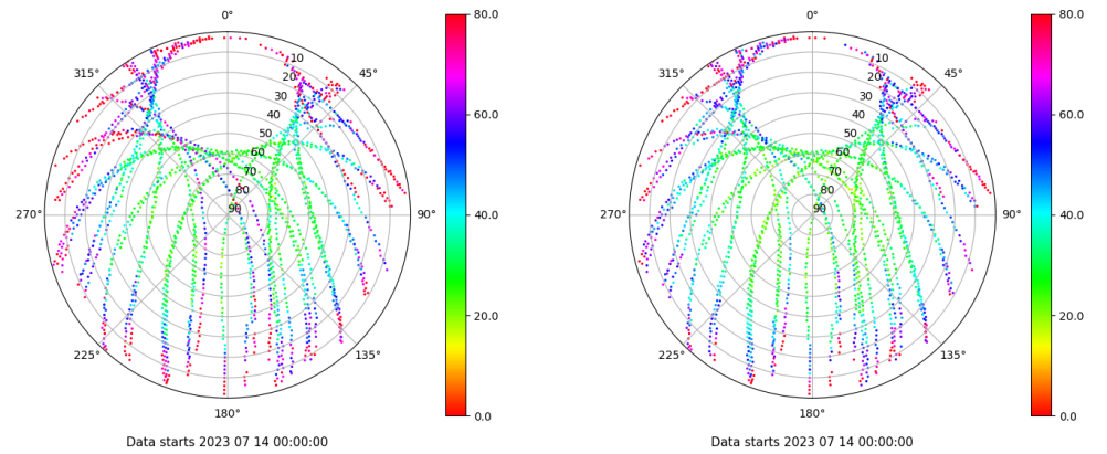
Skyplot for station VIGO. Parameter M1C Data file VIGO00ESP_R_2023195.xtr Skyplot for station VIGO. Parameter M2C Data file VIGO00ESP_R_2023195.xtr
